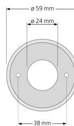
Unteransicht
